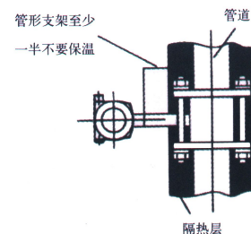
图 13 正确保温图
