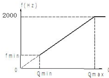
图 12: 脉冲输出频率特性
