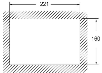
开孔尺寸
